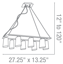
64048 Thea Cable Pendant 8Lt x 40w Halogen 120v JCD (G-9 Base) Finish BS ORB Glass AMB COB OPL Included 10ft of Cable & Cord CUL Dry
