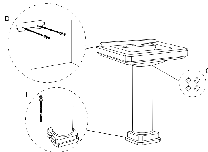
Lavabo sur colonne de 24 po (61cm) Cirtangular®
