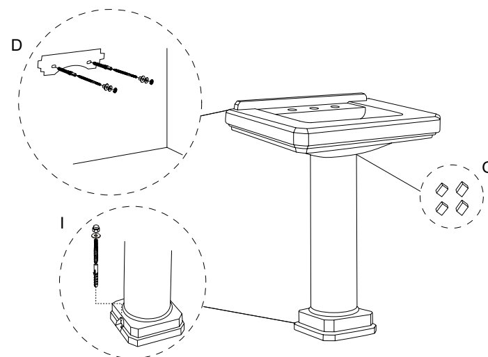
Lavabo tipo pedestal Cirtangular® de 24"
