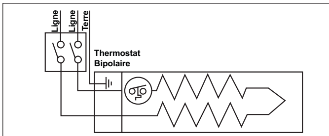
Figure 10 Câblage côté Gauche d'un Thermostat Mural Bipolaire 240 ou 208 volts modèles seulement
