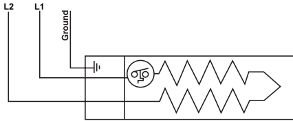
240 or 208 volt models left end wiring
