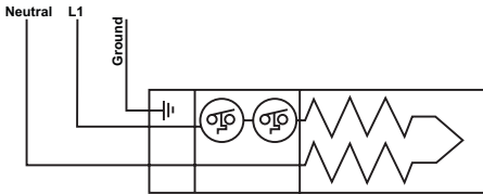
120 volt models left end wiring
