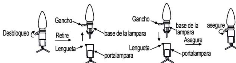
Fig.1 Desbloquee y retire la lámpara quemada
