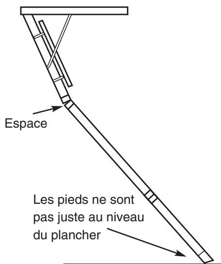
Section inférieure trop longue
