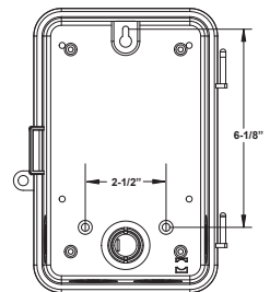
Figure 2 - Vue arrière du boîtier et dimensions des orifices de montage
