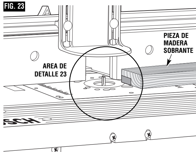
DETALLE 23
