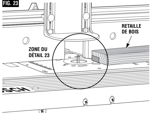
DÉTAIL 23
