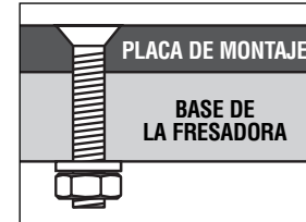
MONTAJE TIPO 2
