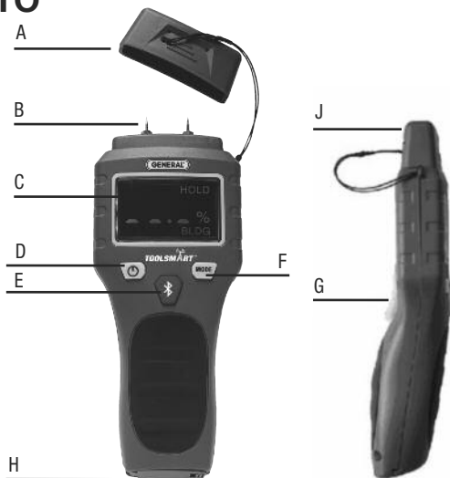
Fig. 1. Controles, indicadores y características físicas del TS06
