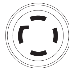
Figura 12 - Receptáculo de 120/240 VAC, 30 Amp
