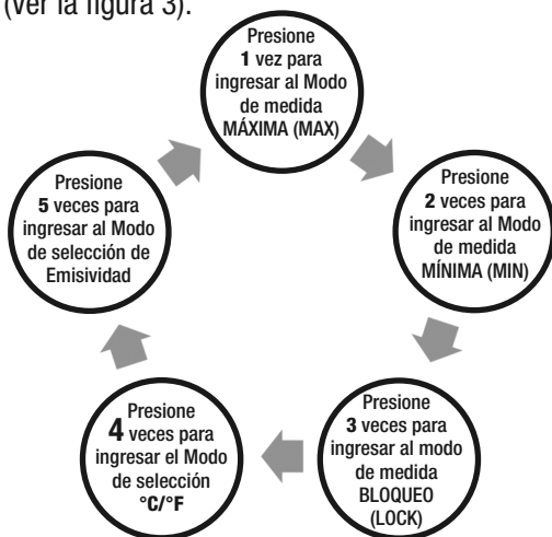
Figura 3. El botón Mode da acceso a la selección de modos y a las 5 medidas avanzadas del IRT105.
