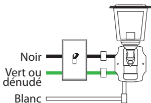
Une lanterne à détecteur de mouvement
