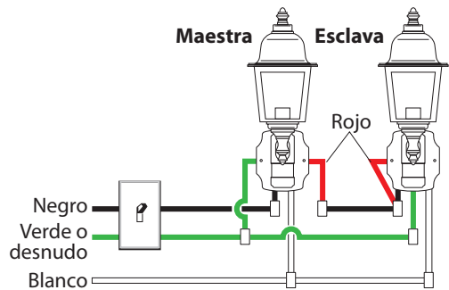
Esquema eléctrico 2
