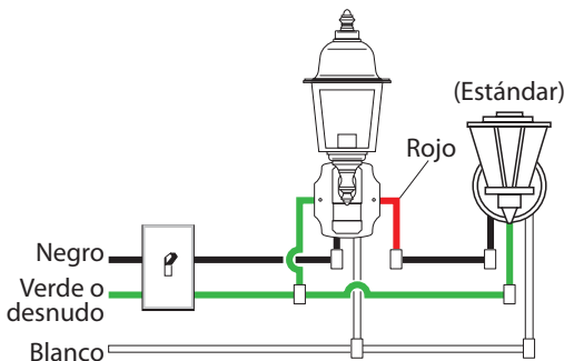
Esquema eléctrico 1
