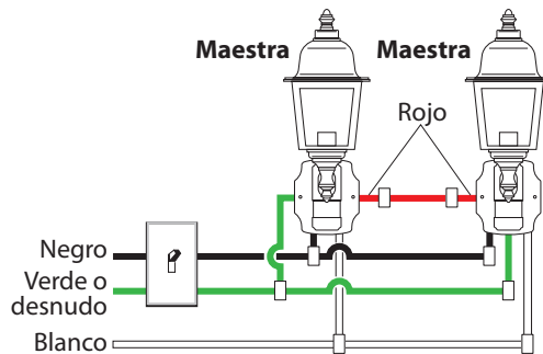
Esquema eléctrico 3
