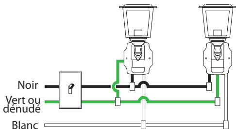
Deux lanternes à détecteur de mouvement
