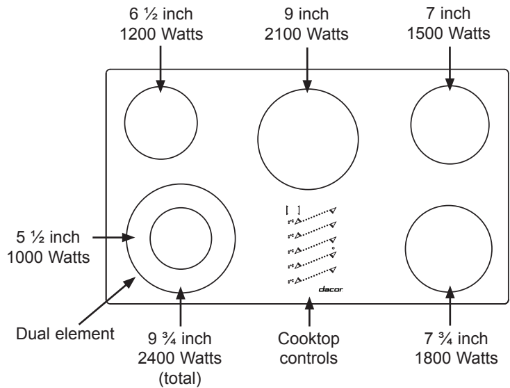
ETT365-2 Cooktop Layout
