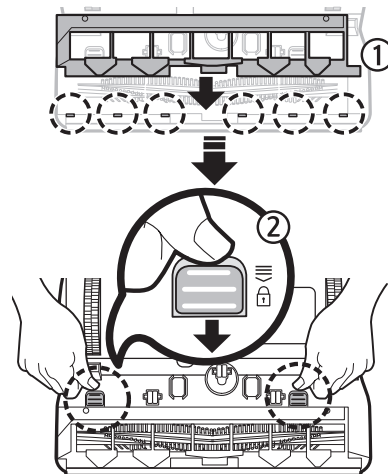
6 Réinstallez le cache de la brosse
