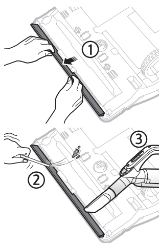
4 Nettoyez le volet obturateur automatique
