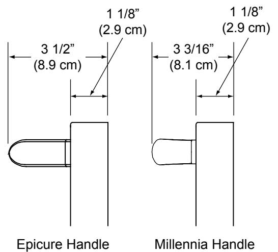
Handle/Front Panel
