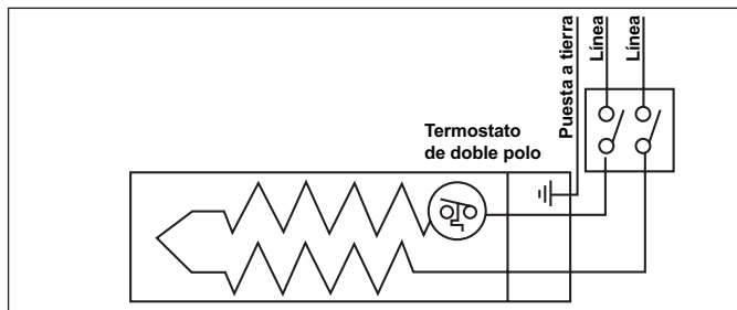
Figura 11 Cableado del extremo Derecho del Termostato Mural de Polo Doble Modelos 240 o 208 voltios solamente
