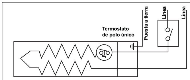
Figura 9 Cableado del extremo Derecho del Termostato Mural de Polo Único Modelos 120, 240 o 208 voltios
