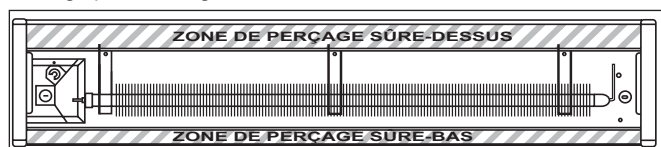
Zones de perçage; câblage par le côté gauche illustré
