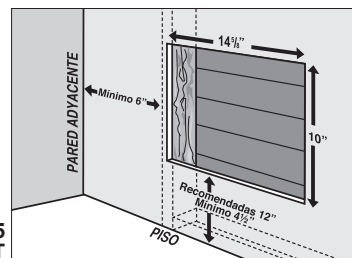
Figura 5 Modelo CST
