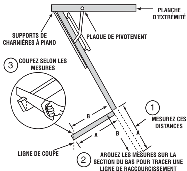
FIGURE 7A - AJUSTEMENT AUX HAUTEURS DE PLAFONDS
