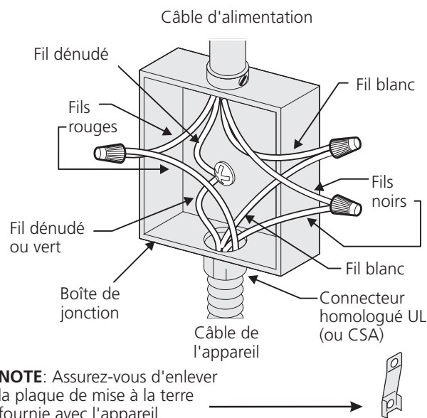
Figure 6 BOÎTE DE JONCTION À 4 FILS - MISE À LA TERRE
