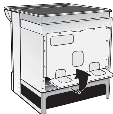
INCLINE AQUÍ LA CUBIERTA DEL ALAMBRE TRASERO PARA TENER ACCEO AL ACOPLAMIENTO ELÉCTRICO
