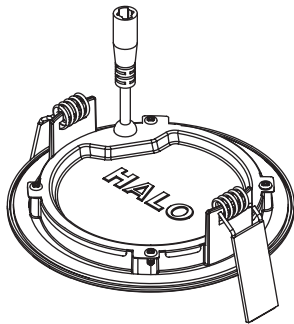
A. HLB and connector, round HLB y conector, rond HLB et connecteur, redondo
