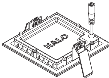
B. HLB and connector, square HLB y conector, carré HLB et connecteur, cuadrado
