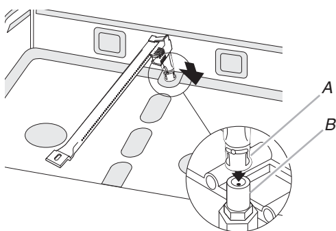
A. Brûleur de cuisson au four B. Gicleur du brûleur de cuisson au four
