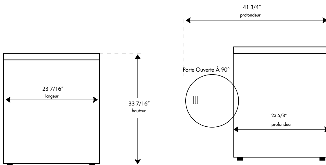
VUE AVANT
