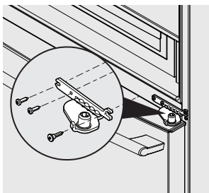
Retirada de la bisagra inferior
