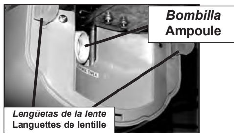
FIG. 9-1 Resbale la lente en la tapa del motor. Faire glisser les lentilles dans le capot du moteur.
