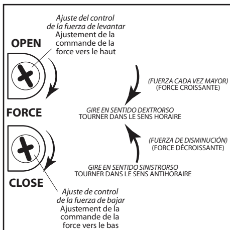
FIG. 6-5 Ajuste de la fuerza de control. Réglage de commande de la force.
