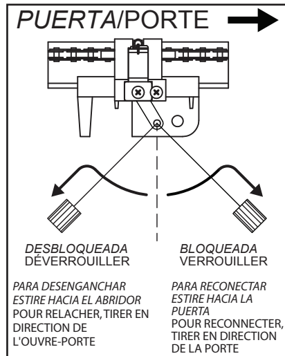
FIG. 6-3 Engranar/ Desengranar bloqueo del corredizo. Engager/Désengager le verrouillage du chariot.
