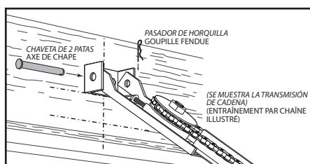
FIG. 2-5 Montaje de riel al soporte del travesaño. Montage du rail sur le support de linéau.
