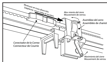
FIG. 6-2 Engrana la cadena al corredizo. Engager la chaîne au chariot.
