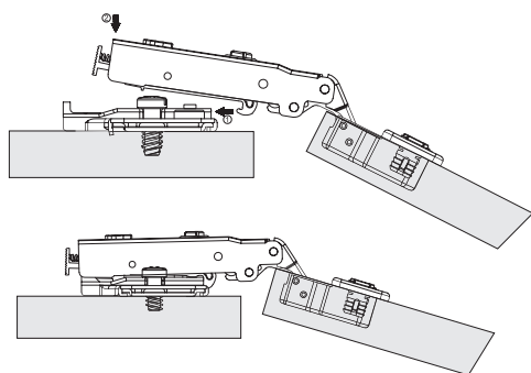
Bisagra de 105°
