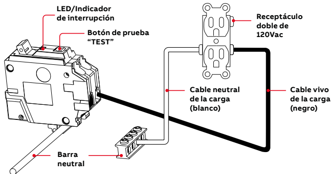
Diagrama de cableado del interruptor de circuito de falla de arco 2
