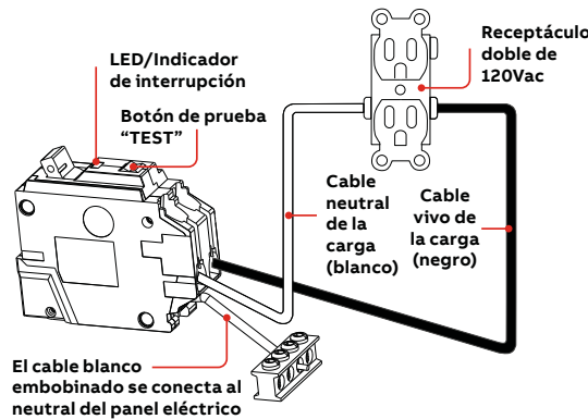
Diagrama de cableado del interruptor de circuito de falla de arco 2
