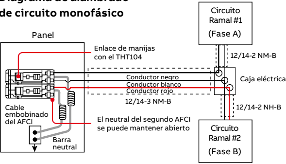
Diagrama de alambrado de circuito monofásico
