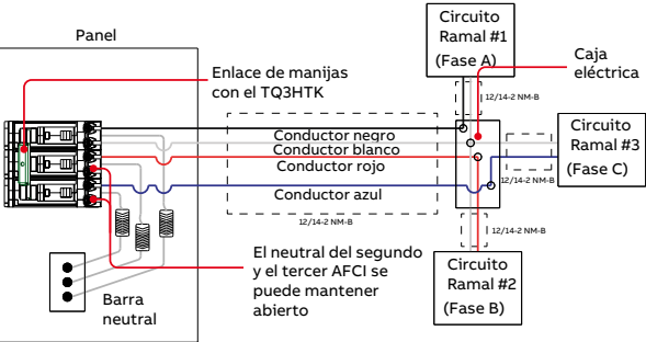
Diagrama de alambrado e circuito trifásico
