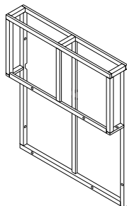
Left back frame (1 pc)
