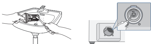
Tapón del filtro de residuos
