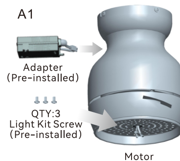
Motor
