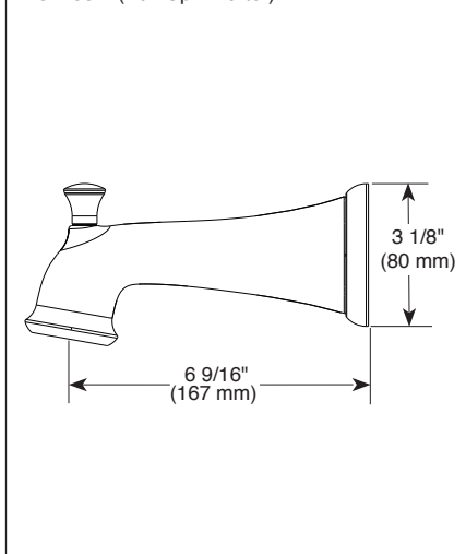
RP52153▲ (Pull-Up Diverter)
