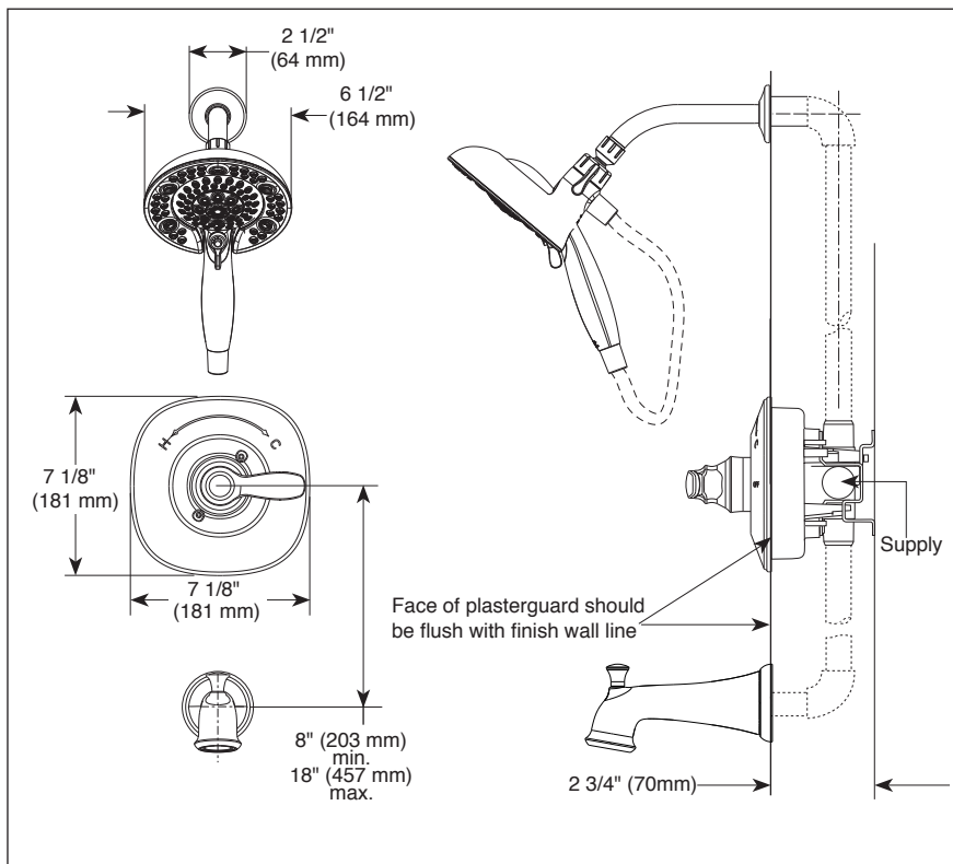
RP52153▲ (Pull-Up Diverter)
