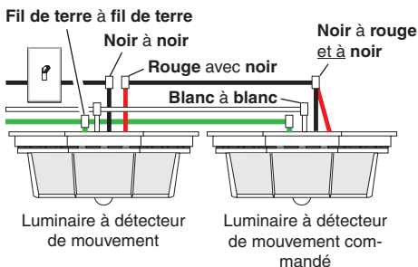
Raccordement d'un luminaire à détecteur de mouvement pour la commande d'un autre luminaire à détecteur de mouvement
