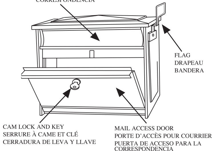
Fig. 1 MAIL SLOT PORTE DE FENTE À COURRIER PUERTA CON RANURA PARA LA CORRESPONDENCIA
