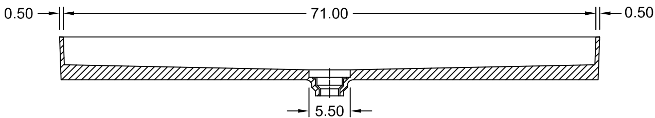
SECTION A-A
