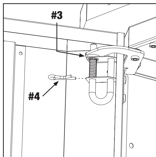
MONTAJE DE CHAVETA
