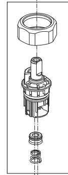
RP71445 Stem Unit Assembly, Seat & Spring, Bonnet Nut Ensamble de la Unidad del Vástago, Asiento, Resorte y Bonete Obturbateur, siège et ressort et écrou à chapeau
