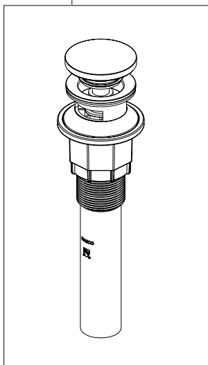
RP100766▲ Push Pop-Up with Overflow Control de rebose para desagües manuales Mécanique à poussoir avec trop-plein
