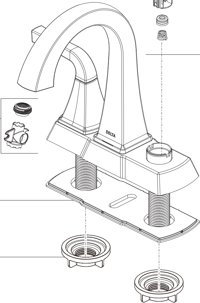
RP101058 1.2 PGM (4.5 L/min) Aerator & Wrench Aireador y Llave Aérateur et Clé
