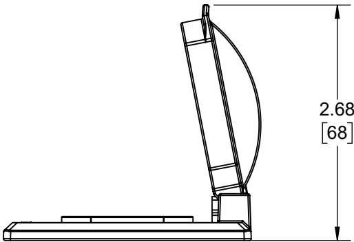
LID OPEN
