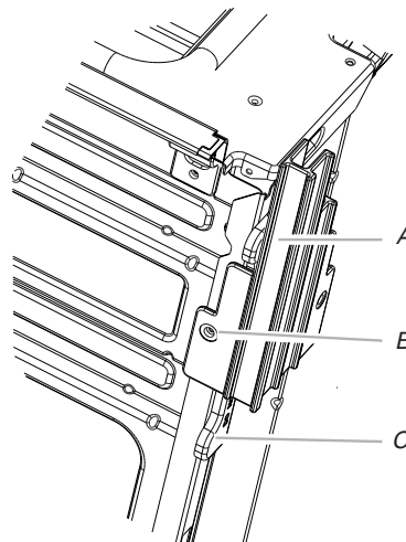
A. Pata delantera B. Tornillo n.º 8-18 x 3/8" (9,5 mm) C. Separador
