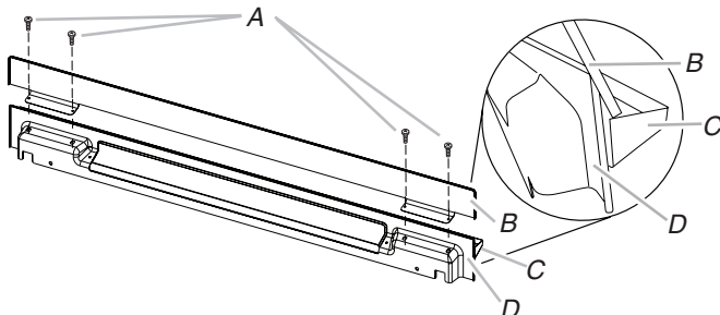
A. Tornillo n.º 8-18 x 1/4" (6,4 mm) B. Borde de ducto de ventilación inferior C. Pieza superior del ducto de ventilación D. Pieza inferior del ducto de ventilación
