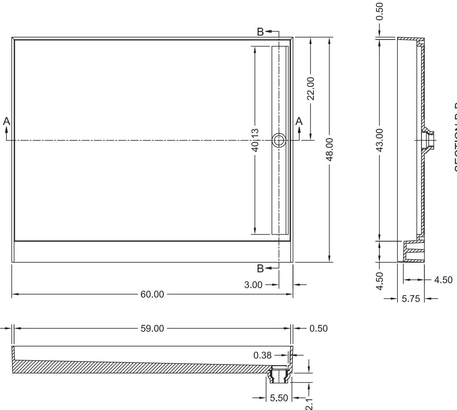
SECTION A-A
