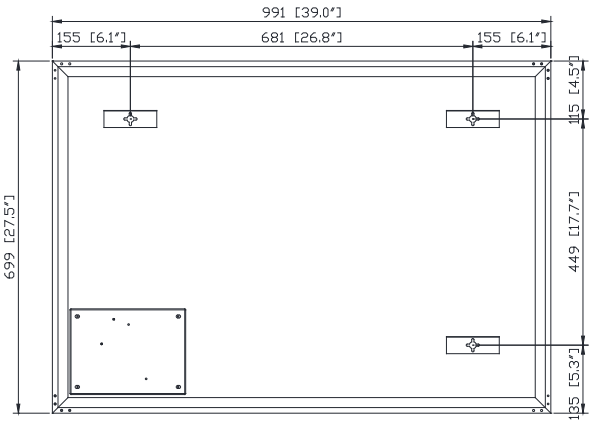
Back / Arrière
