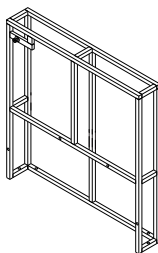
Left frame (1 pc)
