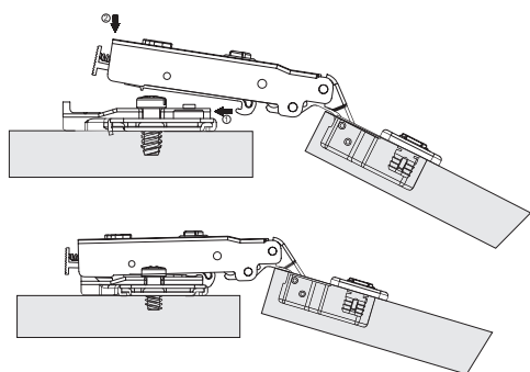
105° Hinge
