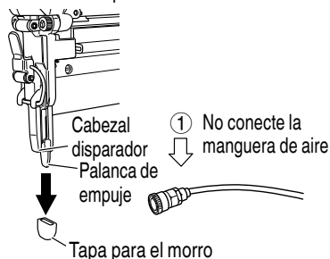
Tapa para el morro
