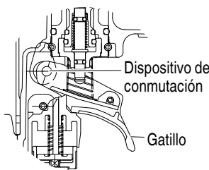
Vista ampliada de la parte de la válvula
