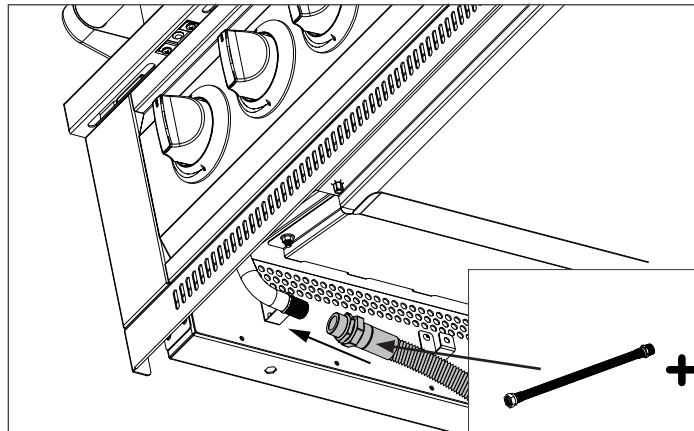
Tuyau d'extension ondulé en métal + PVC Tuyau de gaz naturel en
