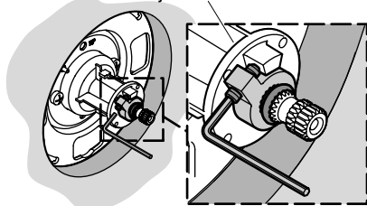
Setscrew Vis de retenue Tornillo de fijación
