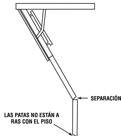
FIGURA 8C INSTALACIÓN INCORRECTA
