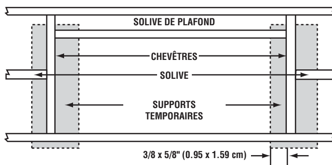
FIGURE 4 – OUVERTURE ENCADRÉE AVEC PLANCHETTES DE SUPPORT TEMPORAIRE PRÊTE À RECEVOIR L'ÉCHELLE
