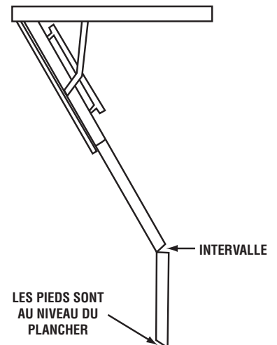
FIGURE 8C - MISE EN PLACE INCORRECTE
