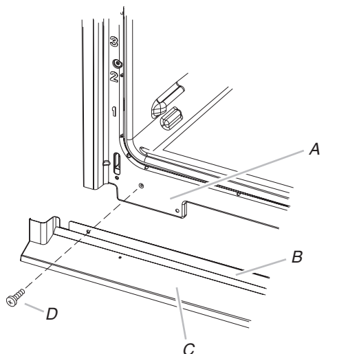
A. Marco del horno B. Lengüeta de ducto de ventilación
