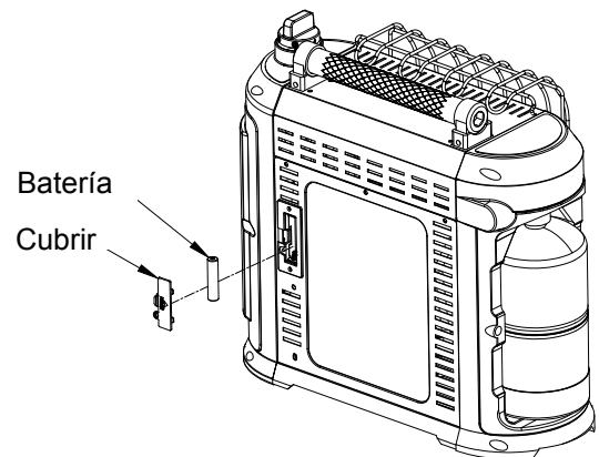
Fig. 3 - Ubicación de la batería para el módulo de chispa
