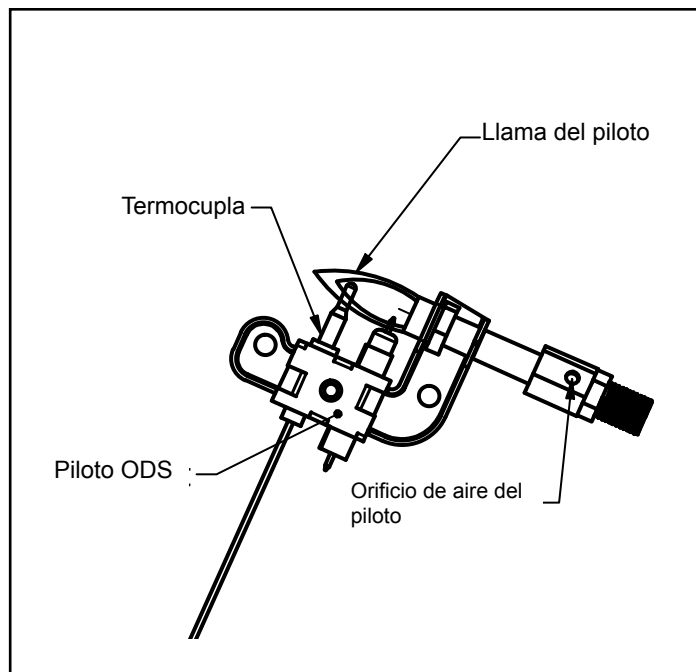
Fig. 5 - Conjunto del piloto
