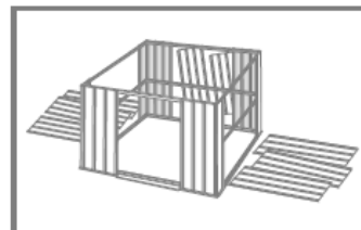
Instalación de los paneles de pared, jambas de puerta y canales
