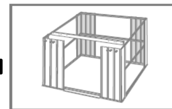
Installation des cadres supérieurs de murs
