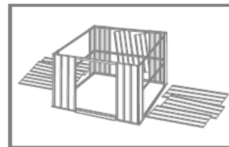
Installation des panneaux de mur, jambages de porte et longerons
