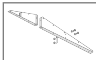
Giebel montieren
