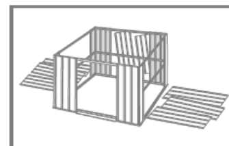
Wandbleche, Türpfosten und Randprofile einbauen
