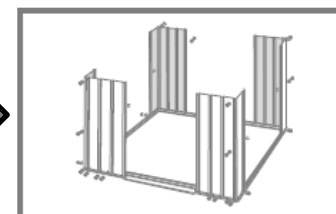
Eckbleche aufstellen
