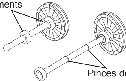
Figure 5 : Ensemble d'arbre de ventilateur
