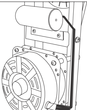
Figura 4: Ensamblaje del capacitor
