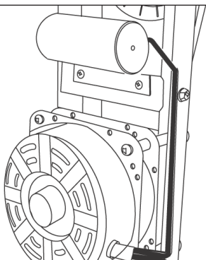
Figure 4 : Ensemble de condensateur
