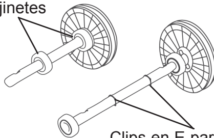
Figura 5: Ensamblaje del eje del ventilador
